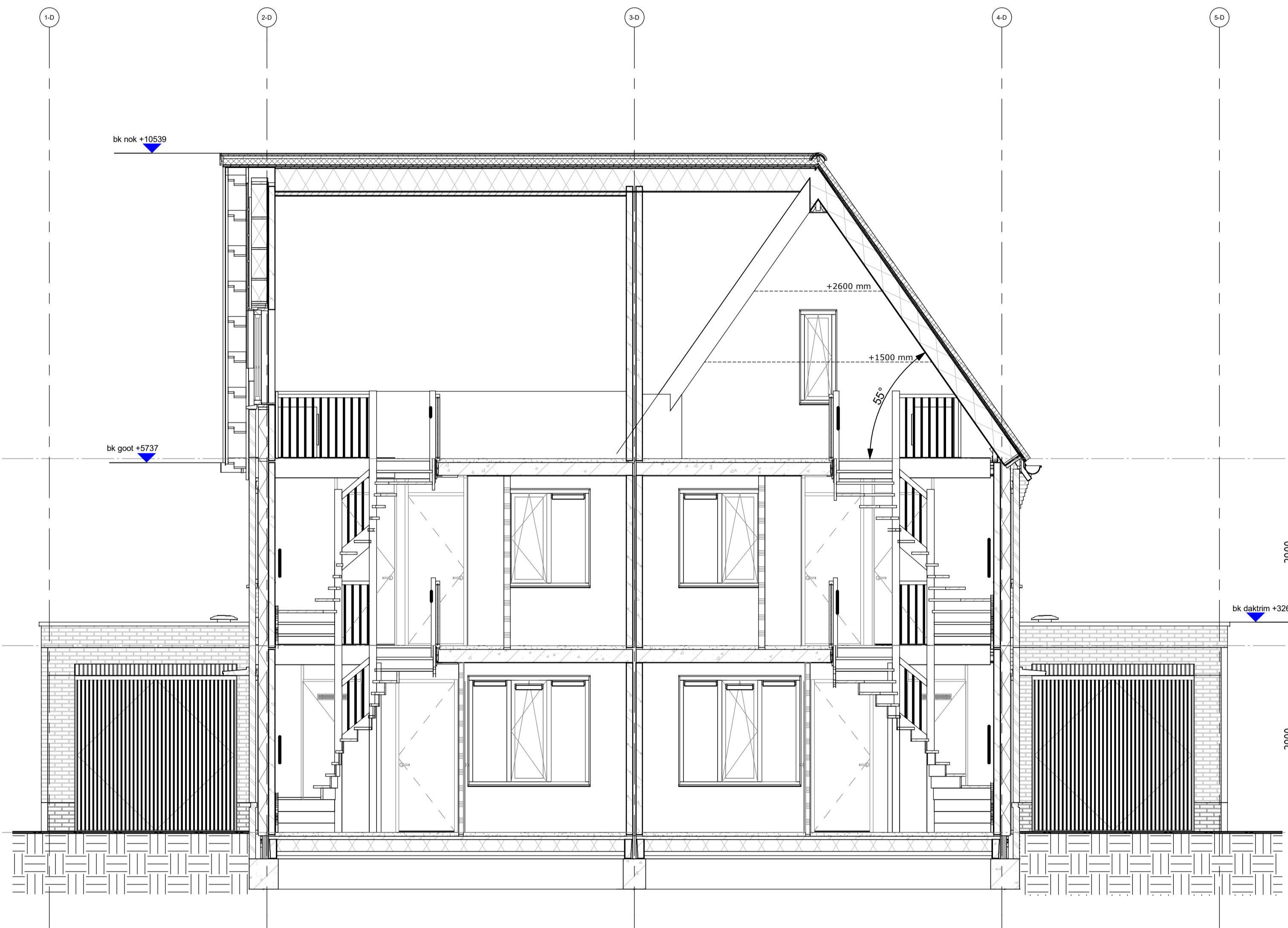
Langsdoorsnede
