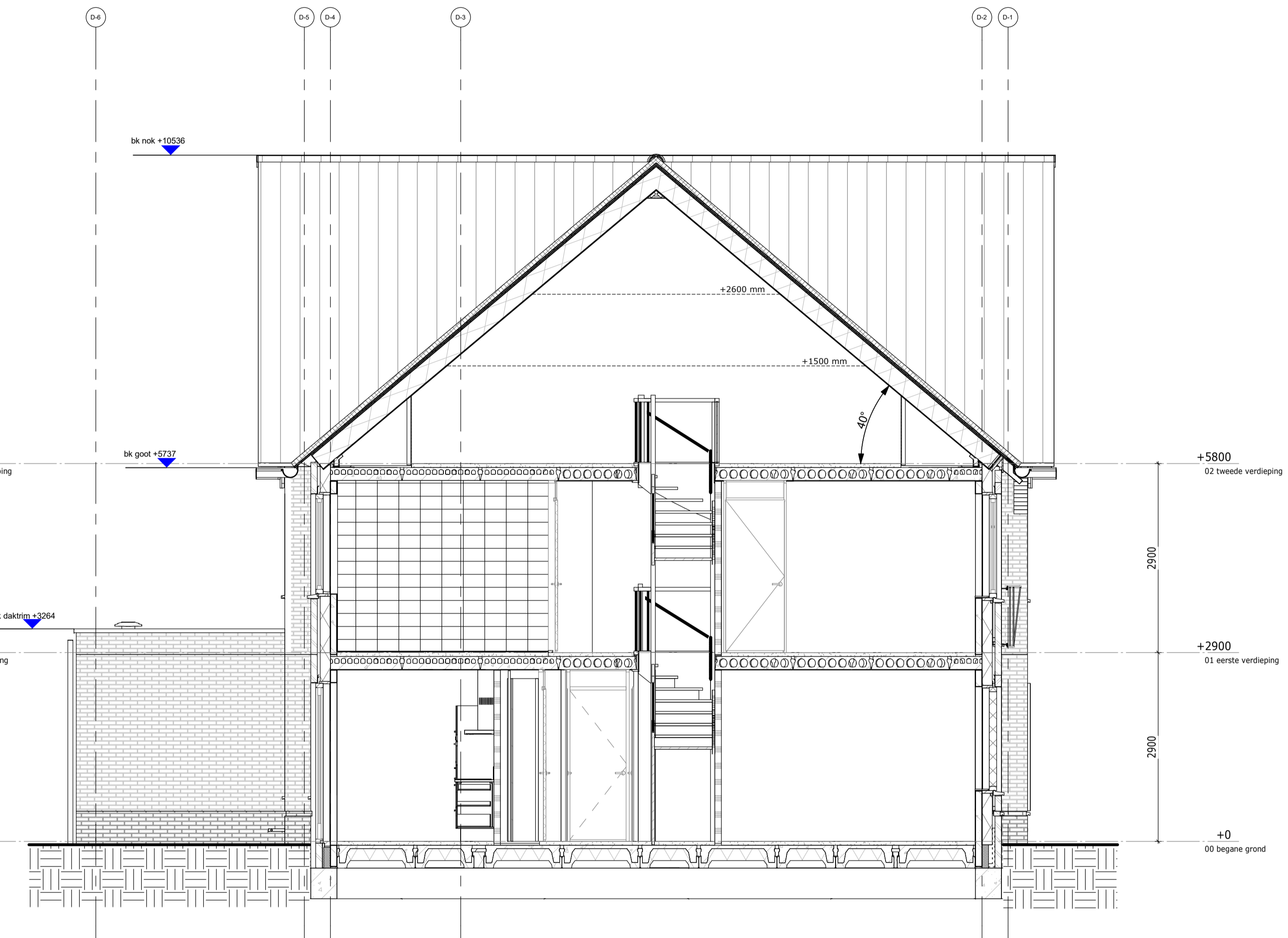
Dwarsdoorsnede
