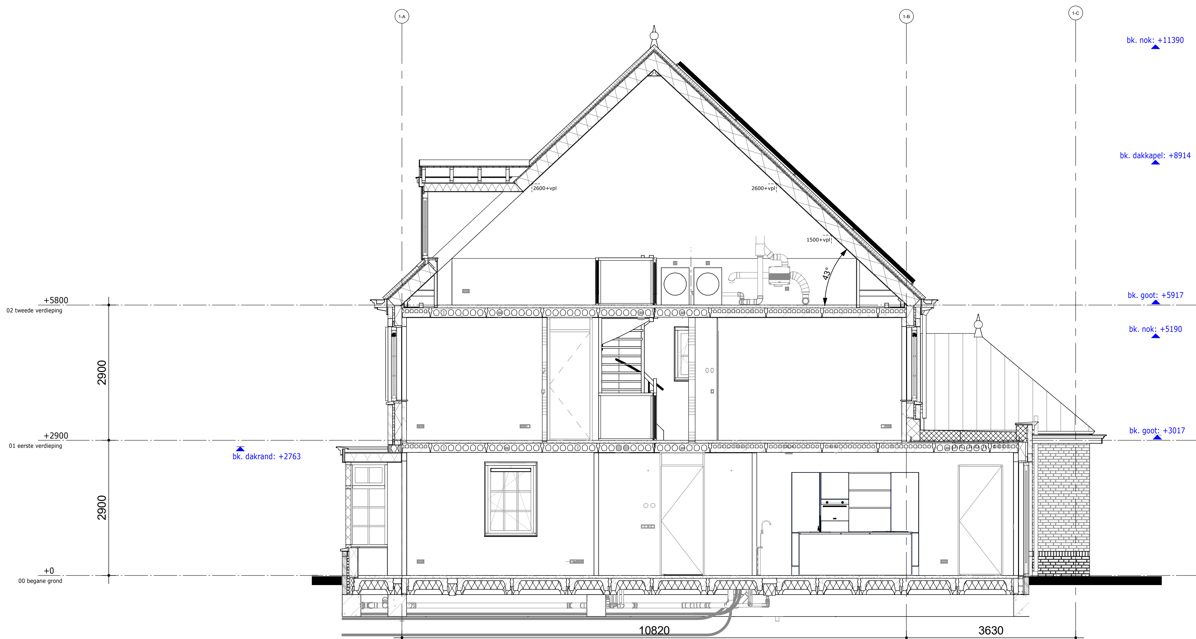
Langsdoorsnede
