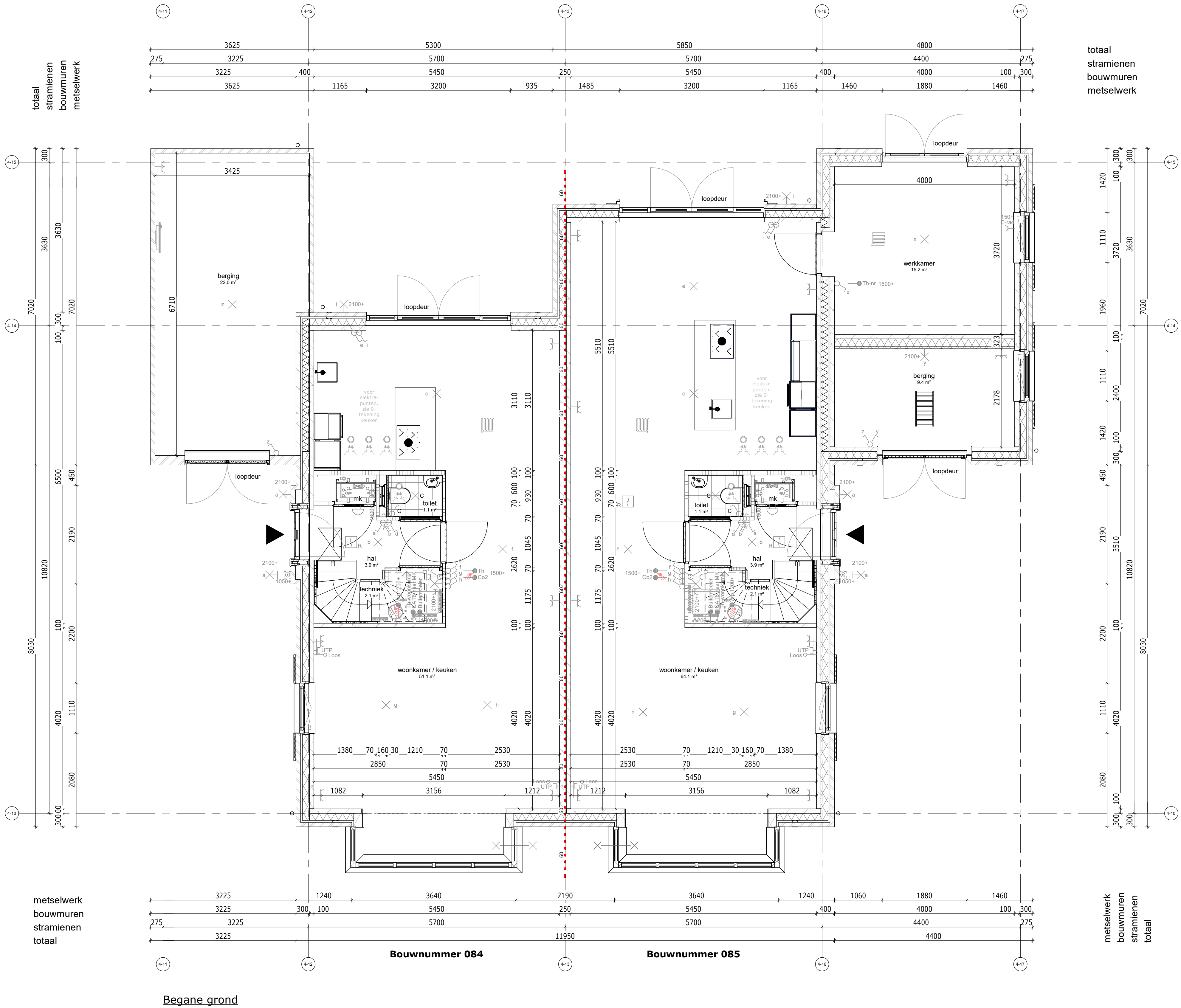
Begane grond
