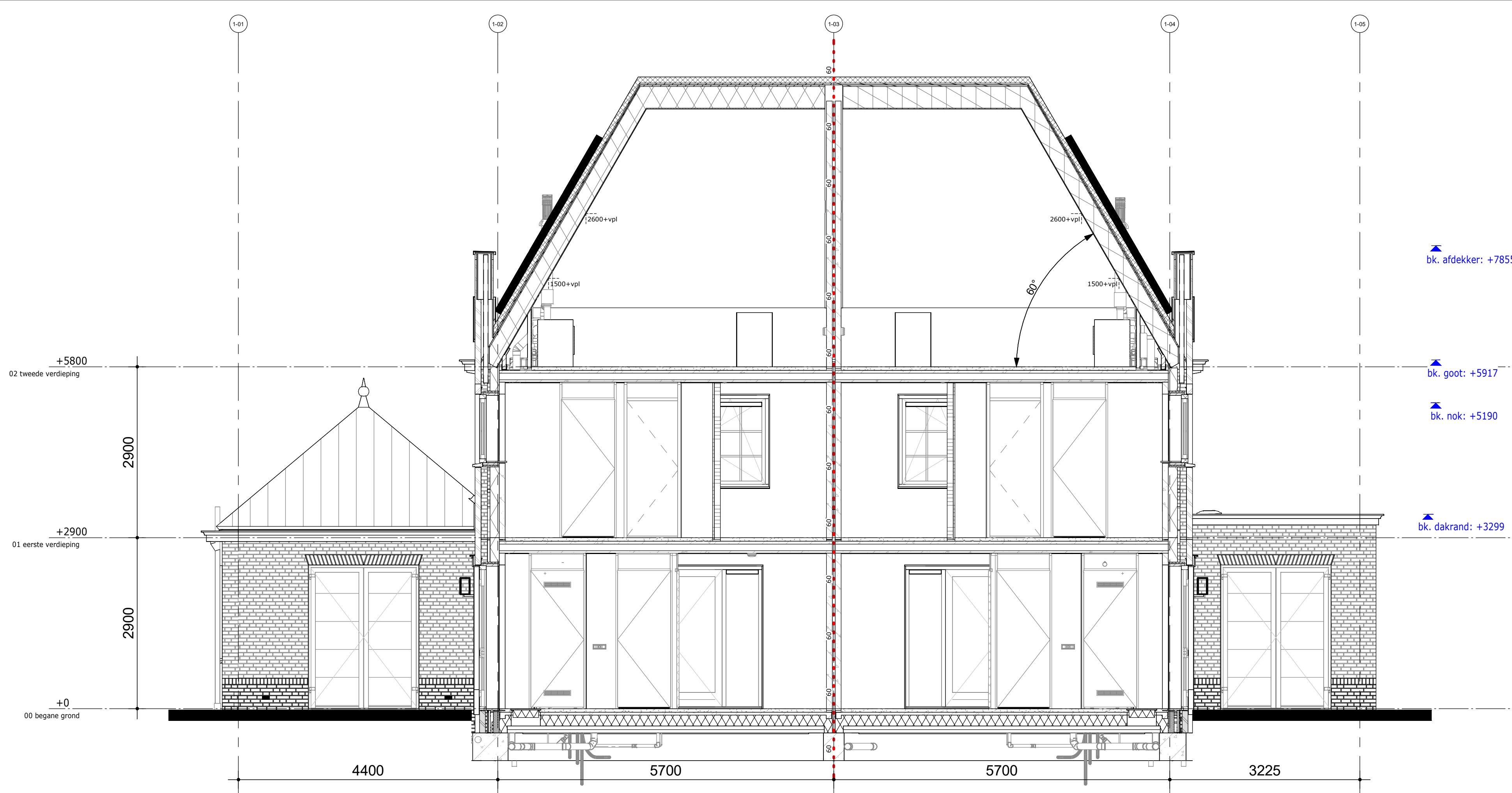
Dwarsdoorsnede
