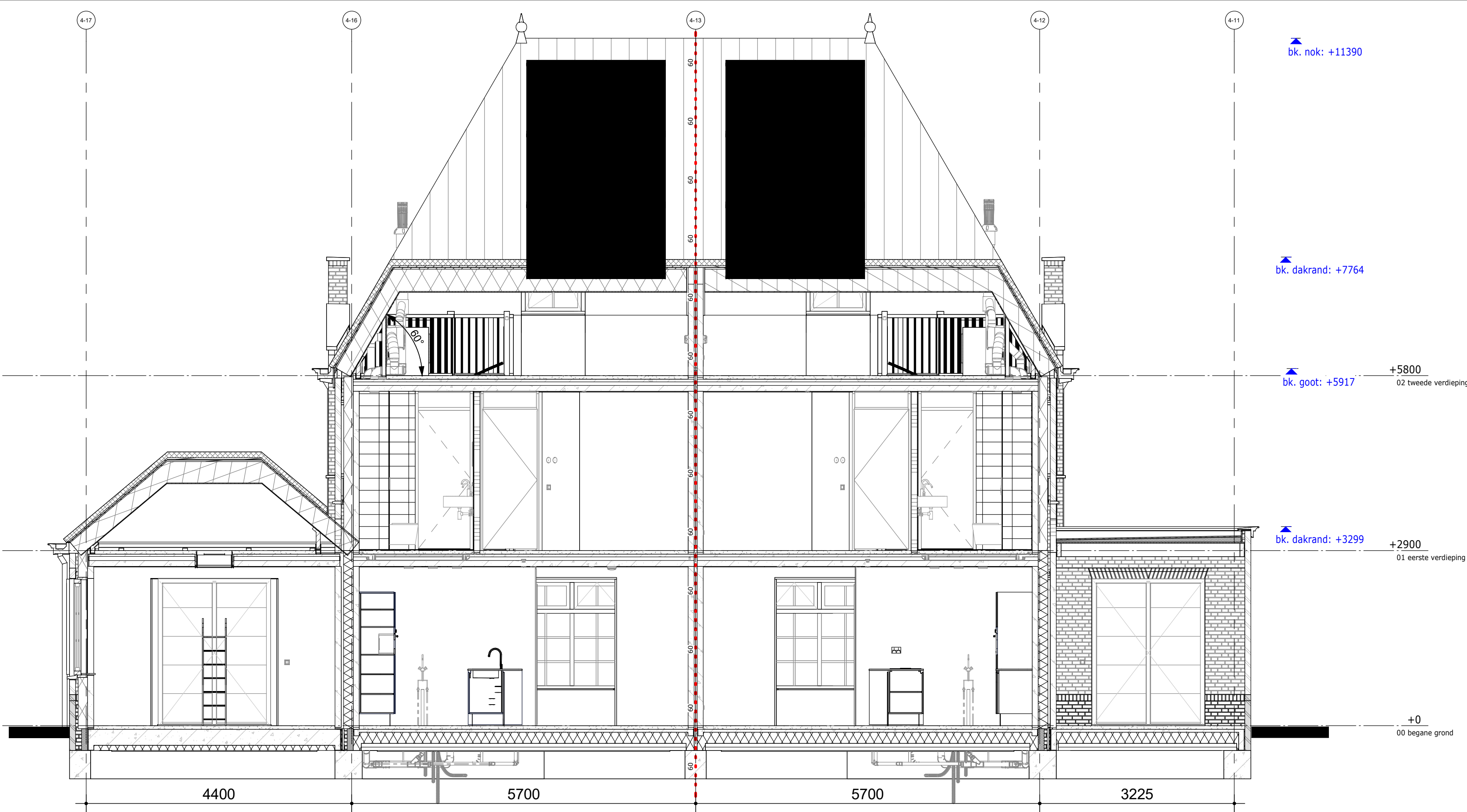
Dwarsdoorsnede
