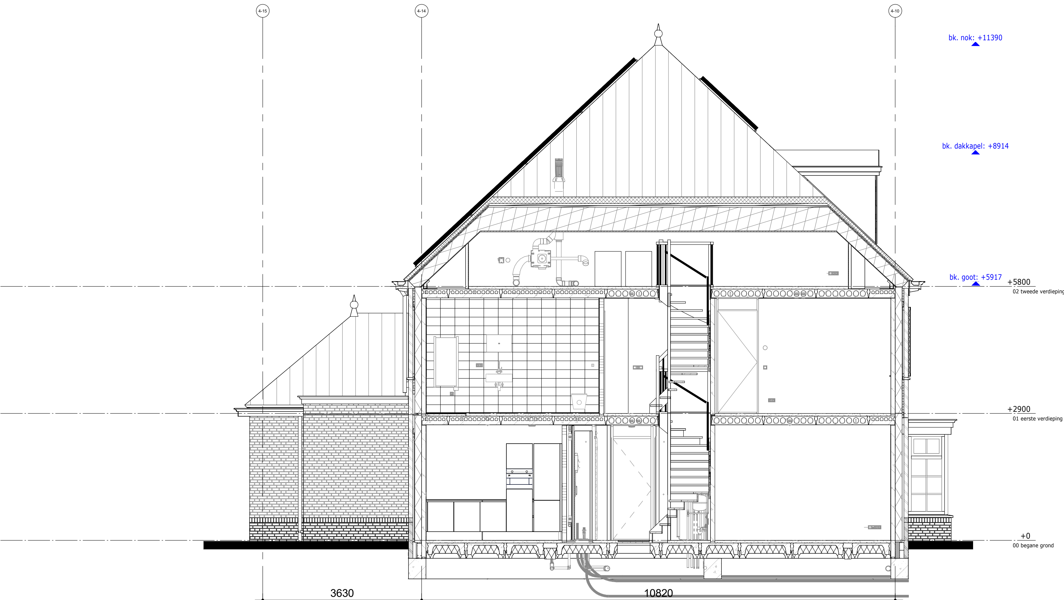
Langsdoorsnede
