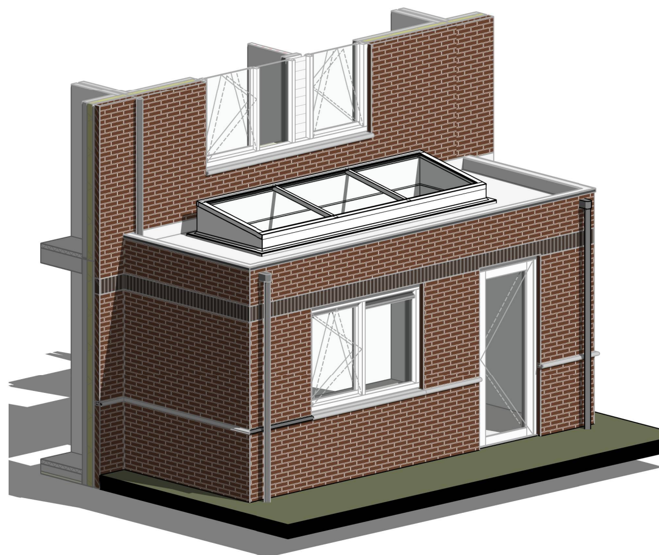
9500900_3D Lichtstraat
