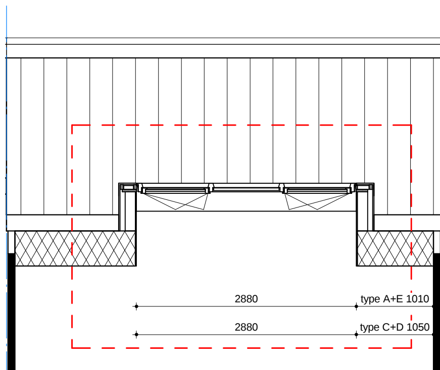
9312500_dakkapel-2880
