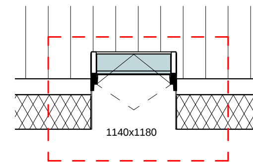
9500600 plaatsen dakraam
