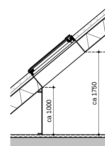
9500600 Doorsnede dakraam
