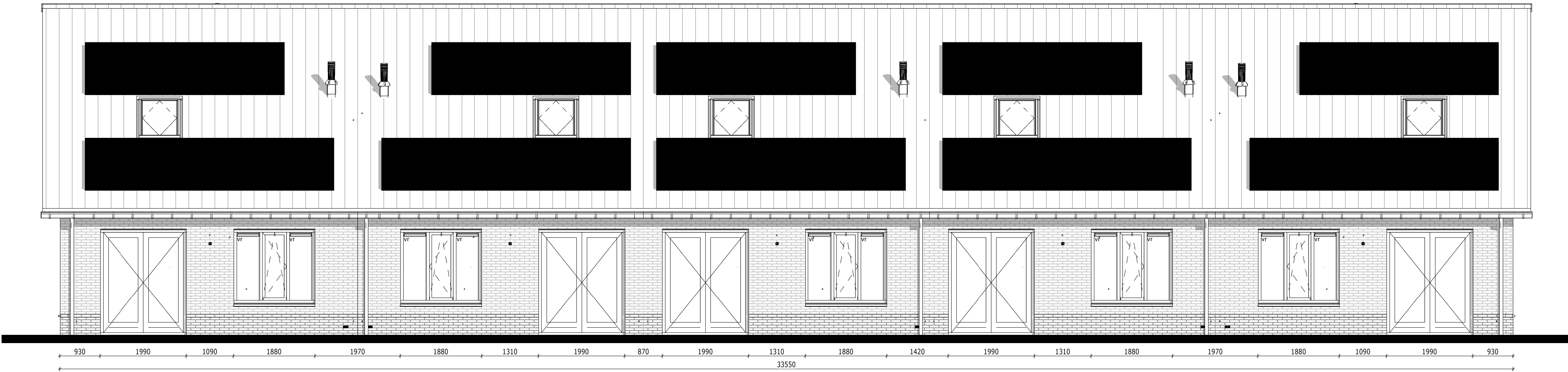
Blok 14 - achtergevel 1 : 50
