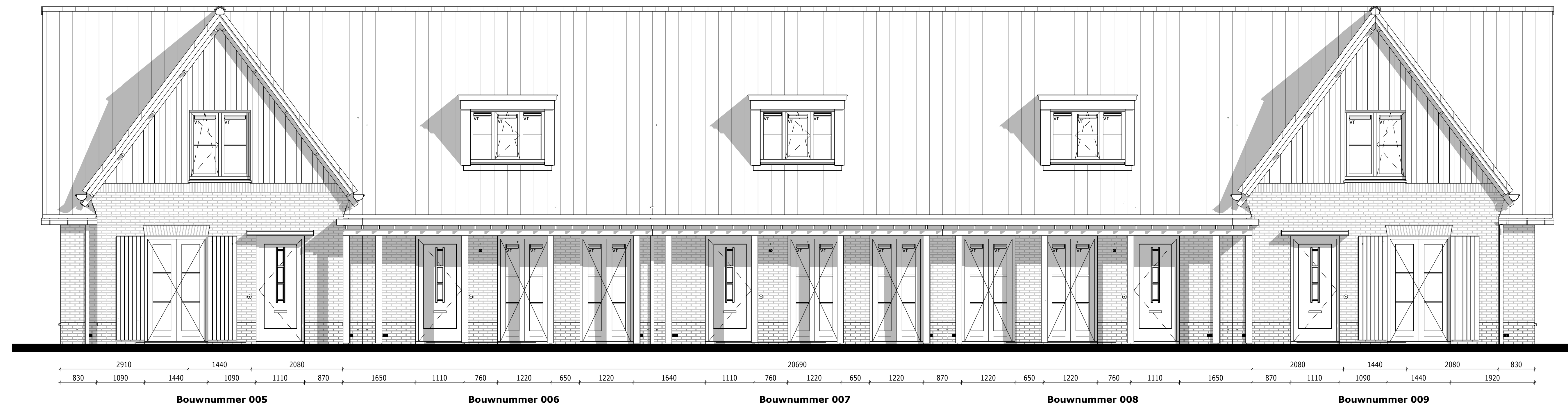
Blok 14 - voorgevel 1 : 50
