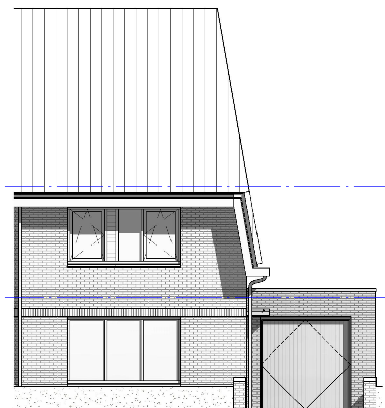
Voorgevel - bouwnr 01
