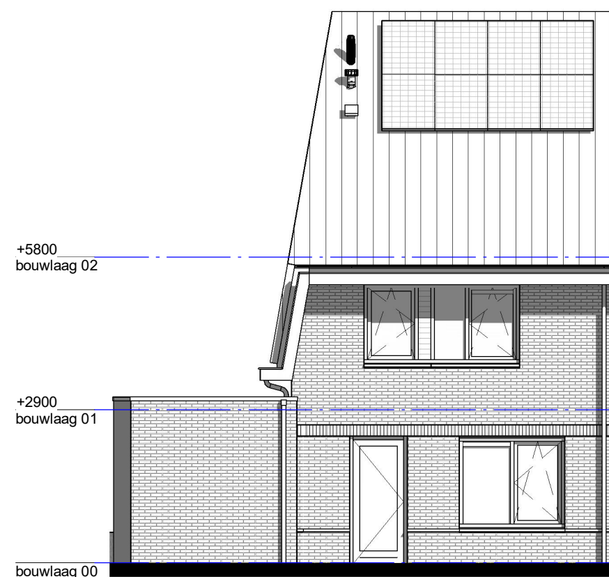
Achtergevel - bouwnr 01
