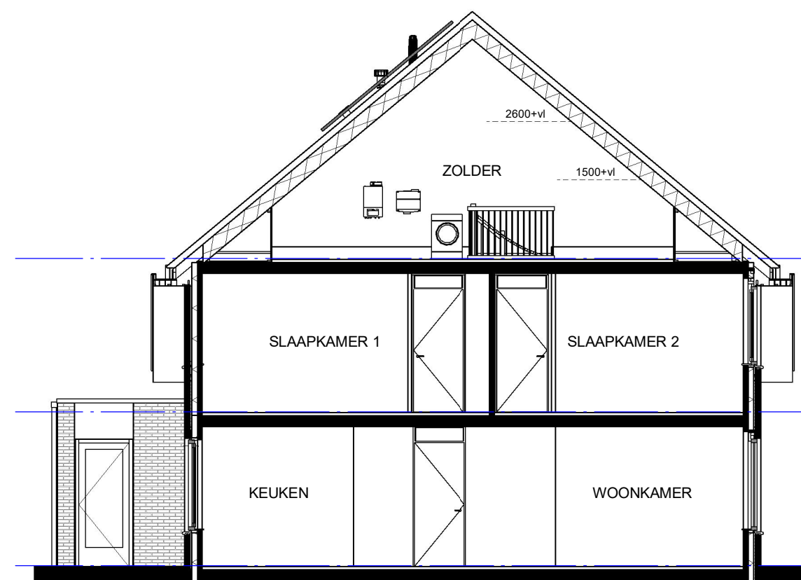
Doorsnede - bouwnr 01
