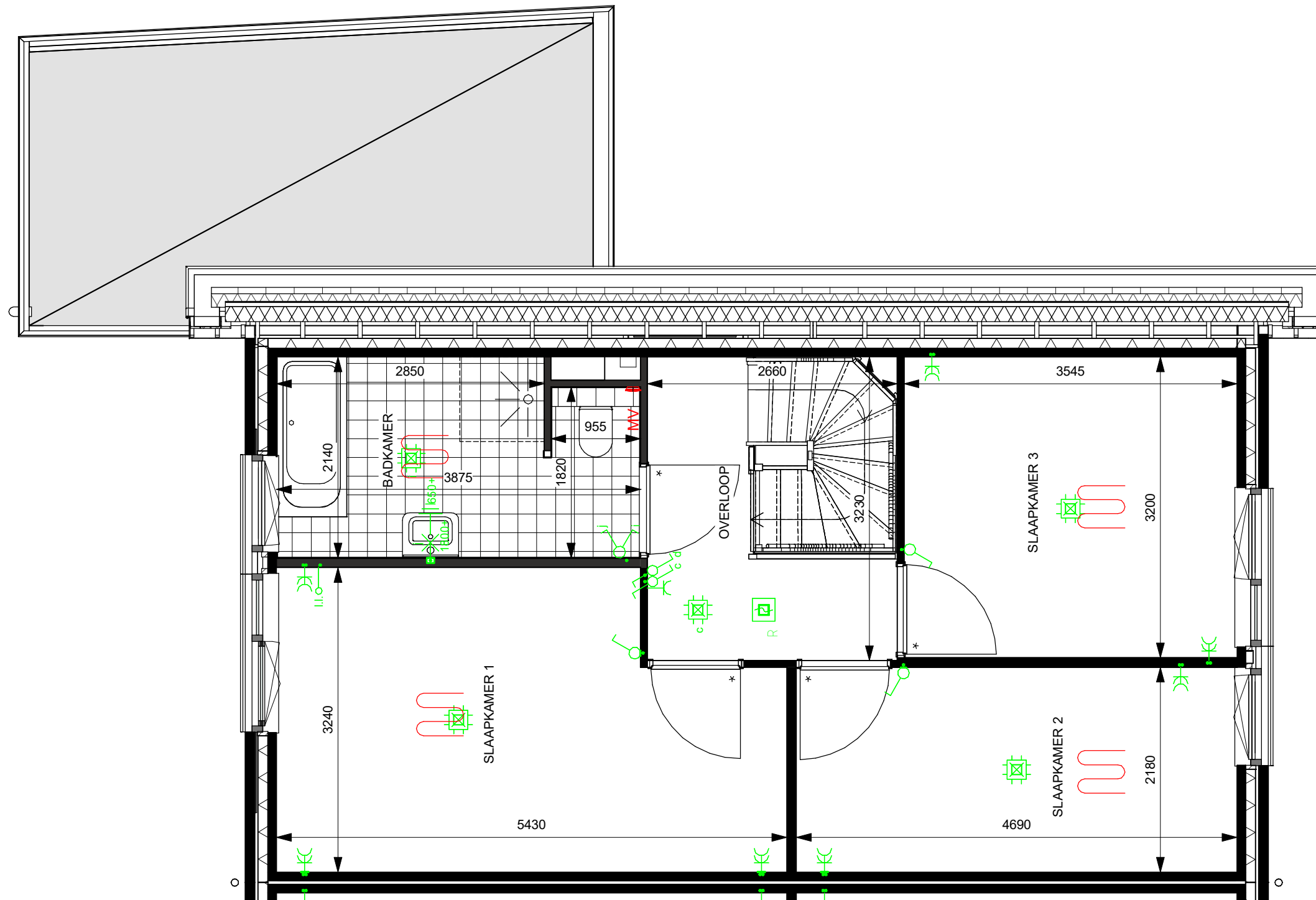
01 bouwlaag - bouwnr 01
