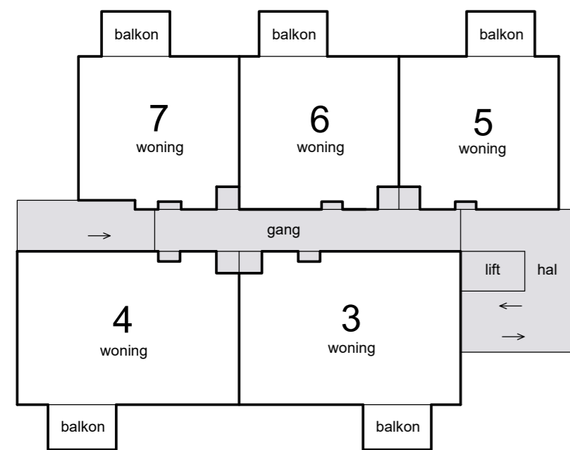
1e verdieping
