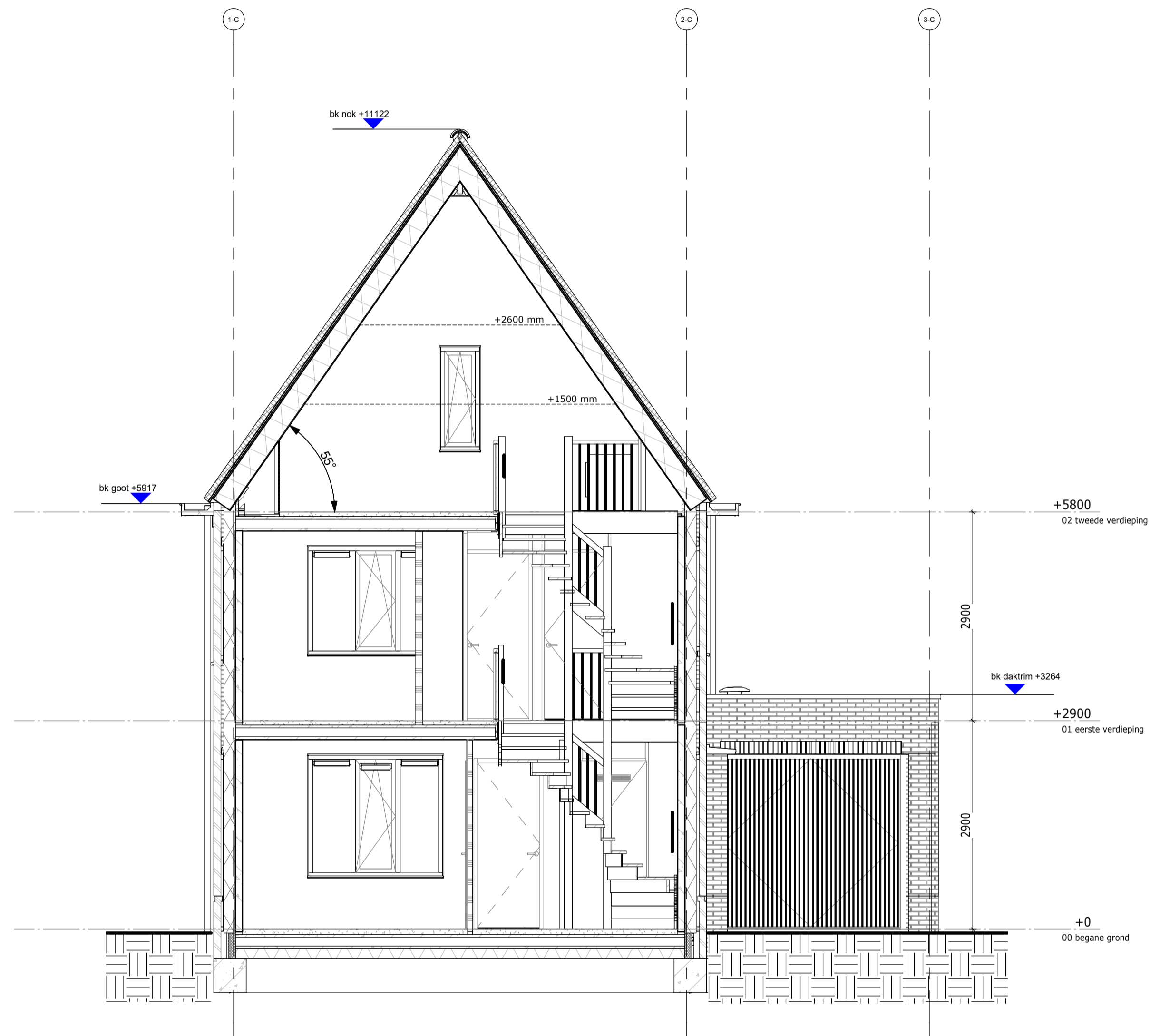
Dwarsdoorsnede
