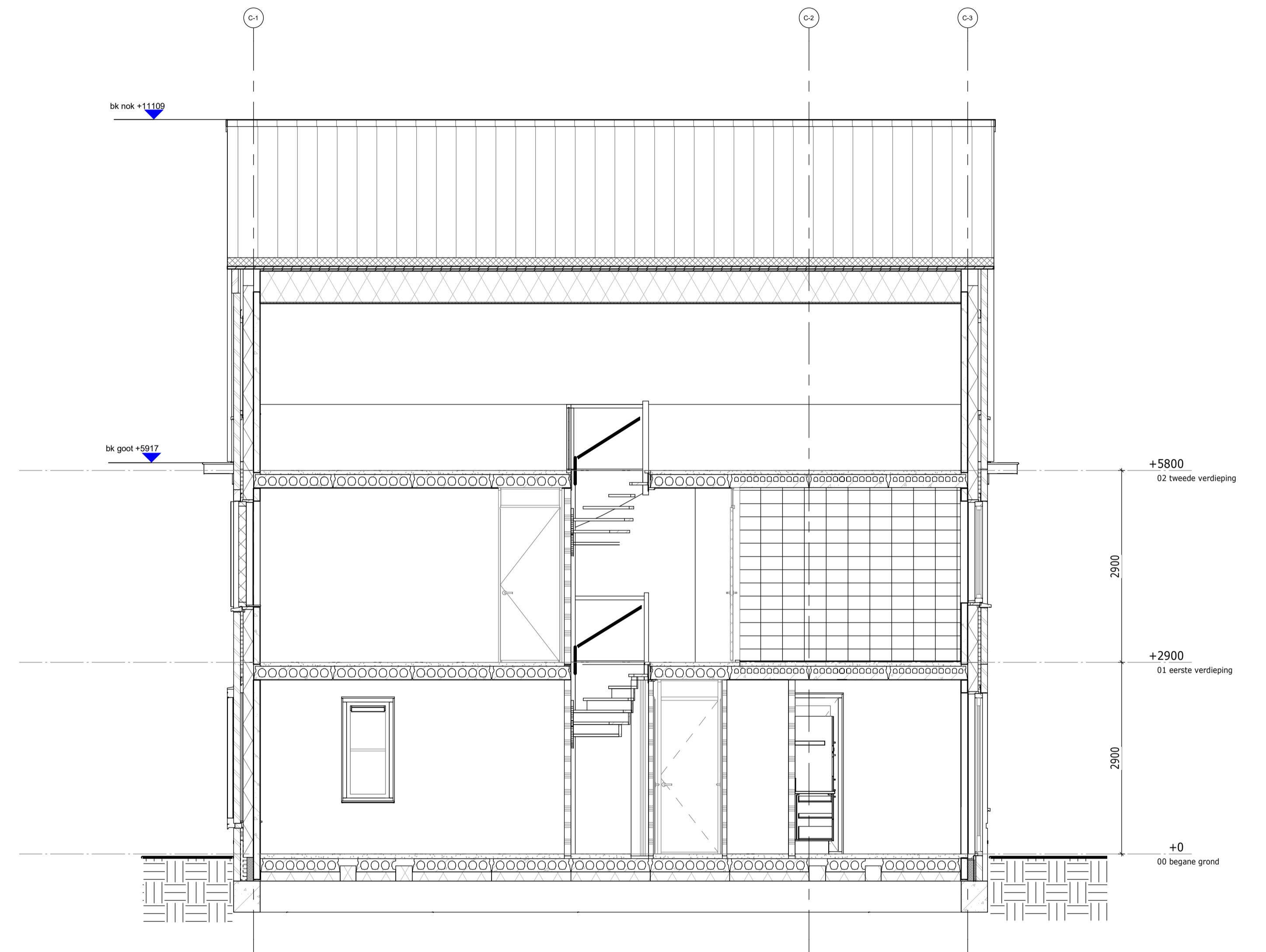
Langsdoorsnede
